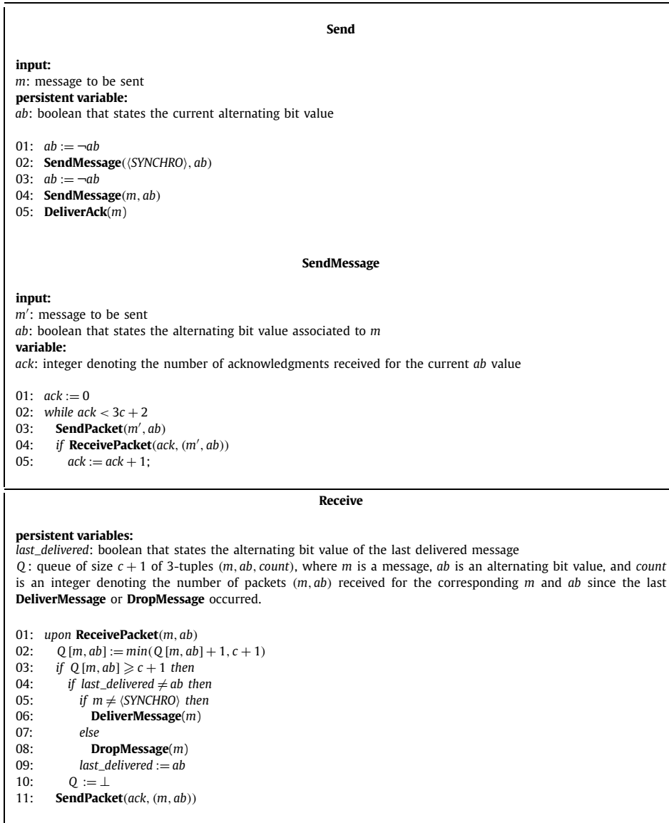
Fig. 2. SDL , a (0, 1, 1, 1)-Stabilizing Data-Link protocol.
